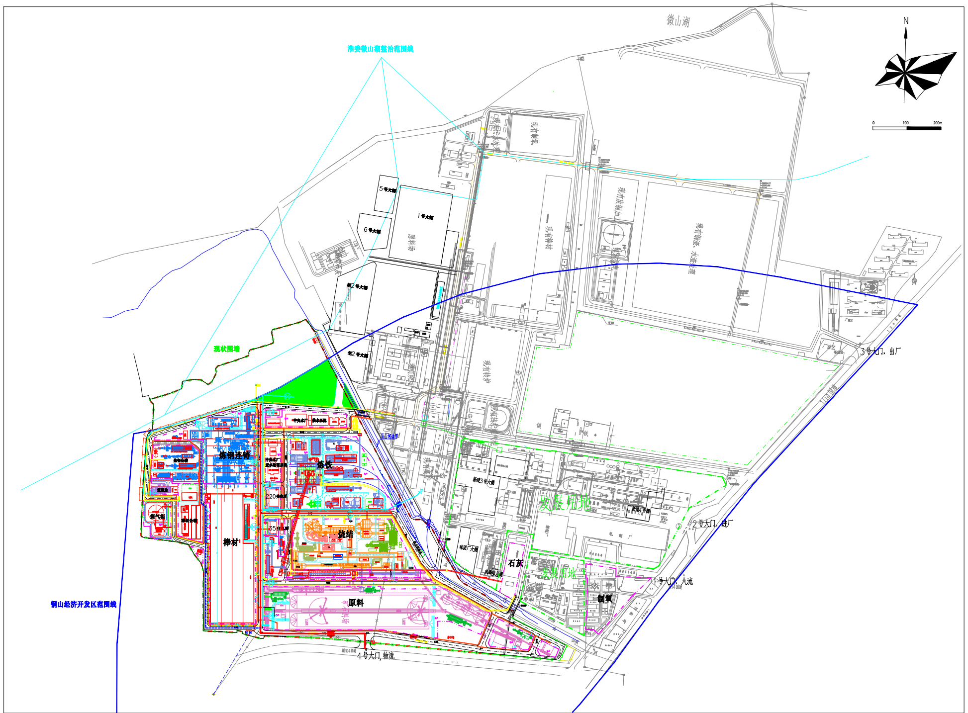
图3.3-4 (1) 本工程厂平面布置图
